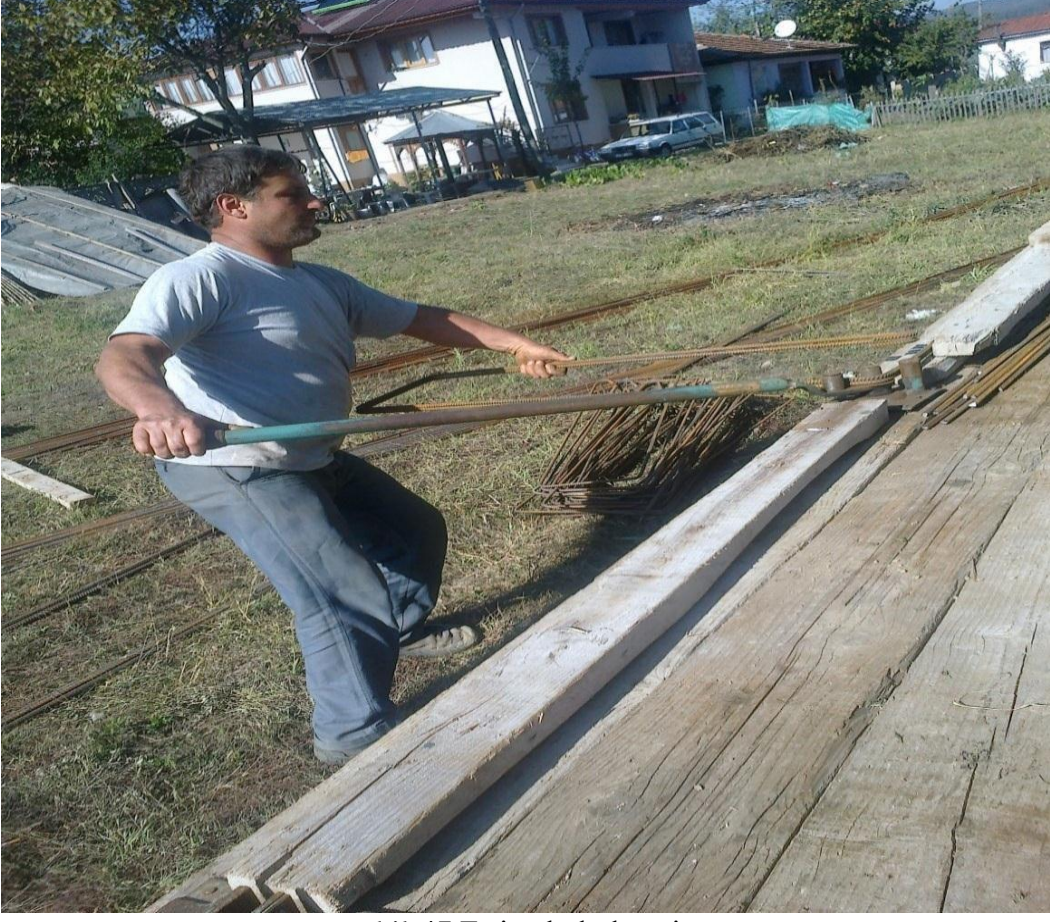
ğekil-47 Etriye bükülmesi
